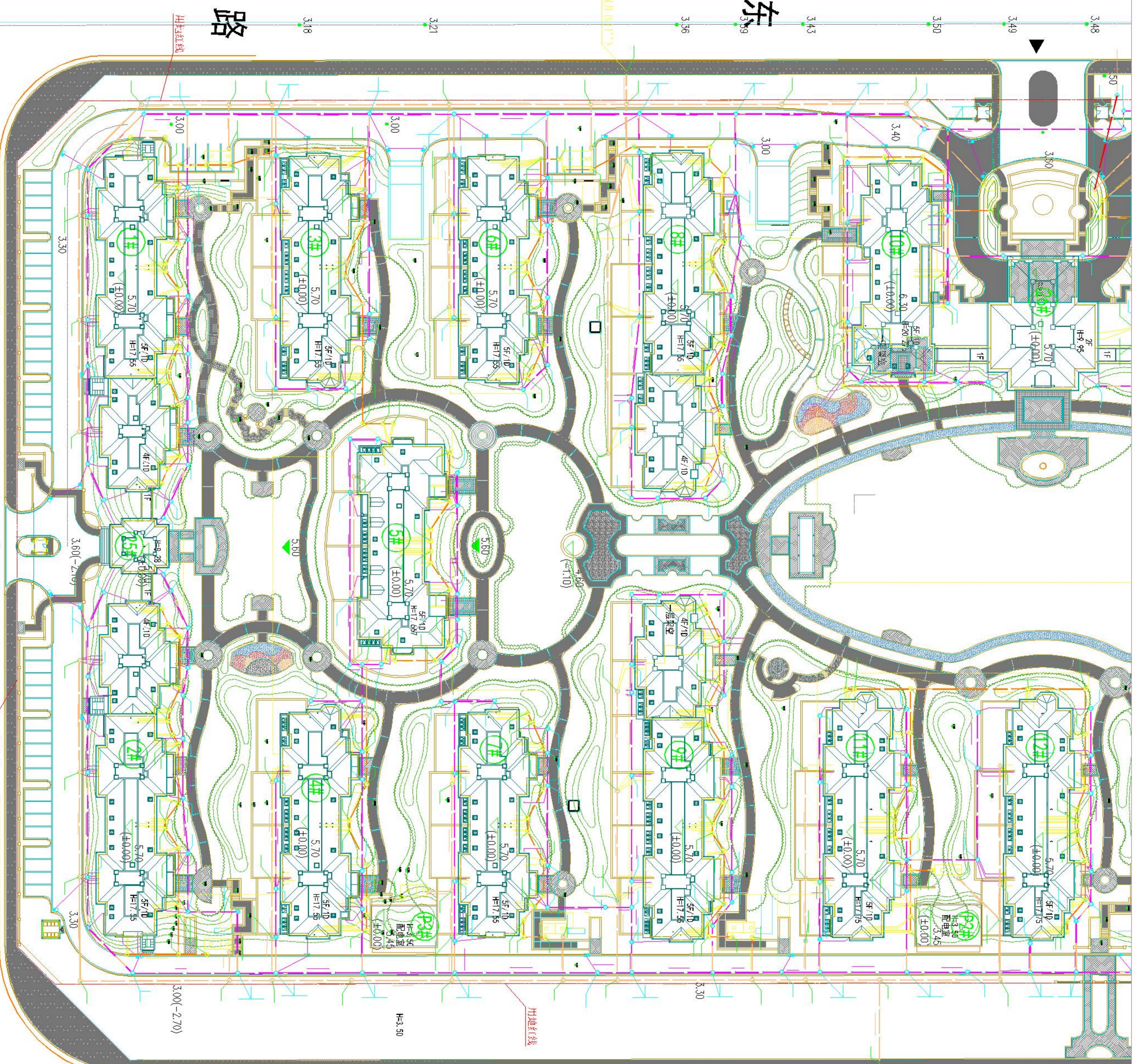
室外排水管道平面图二
